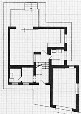
PŘÍZEMÍ GROUND FLOOR
