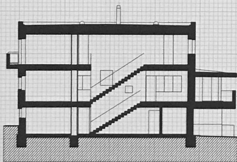
ŘEZ SECTION
